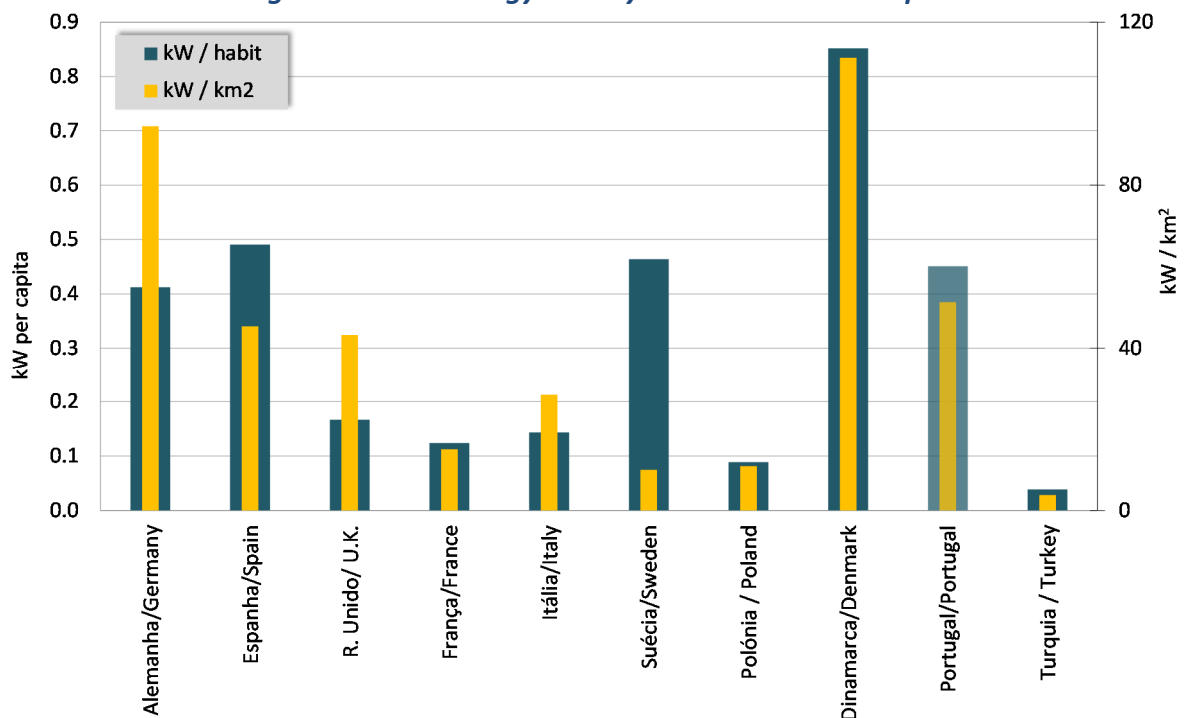
Figura 4: Índices de densidade 2015 - Europa Figure 4: Wind energy density indexes 2015 - Europe
