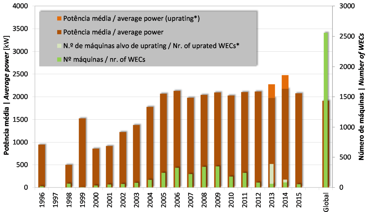
Figura 16: Número de aerogeradores e potência unitária média 1996-2015 Figure 16: Number of WECs and mean rated power 1996-2015
