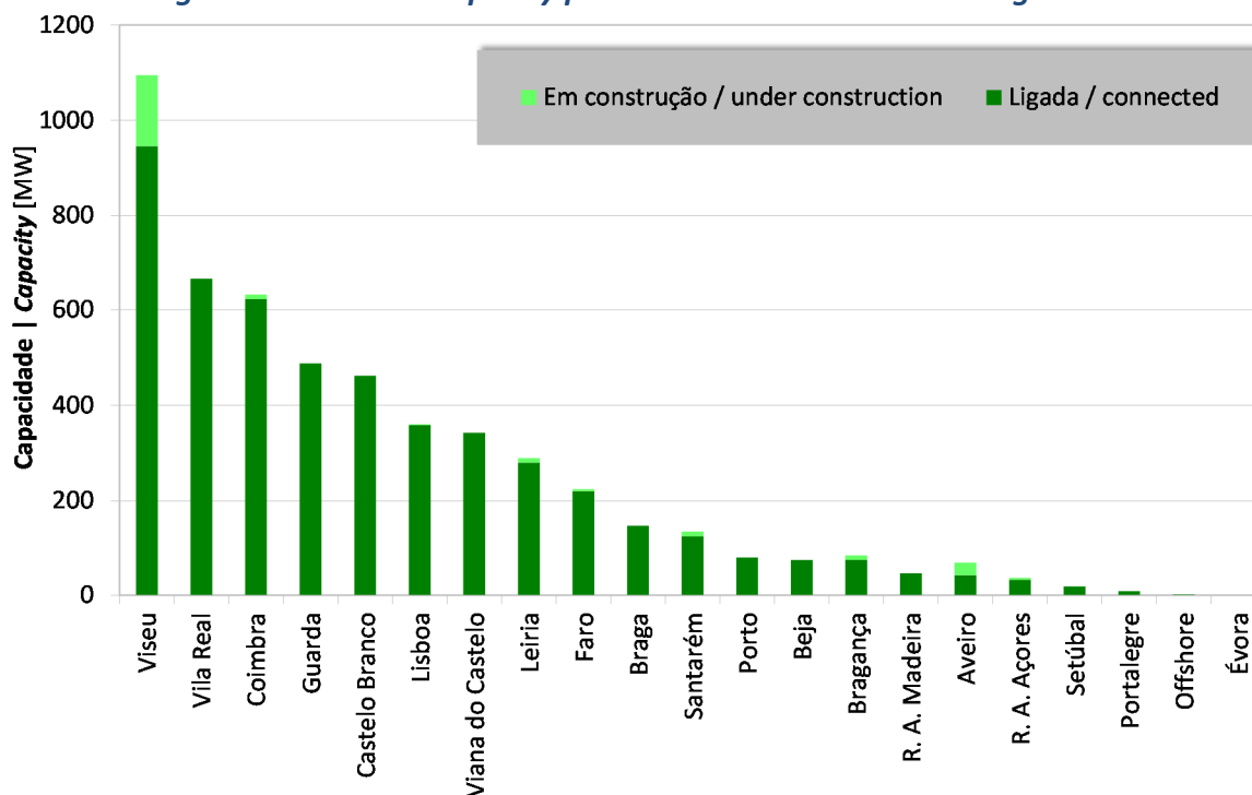
Figura 13: Potência Instalada por Distritos e Regiões Autónomas 2015 Figure 13: Installed capacity per district and autonomous region 2015
