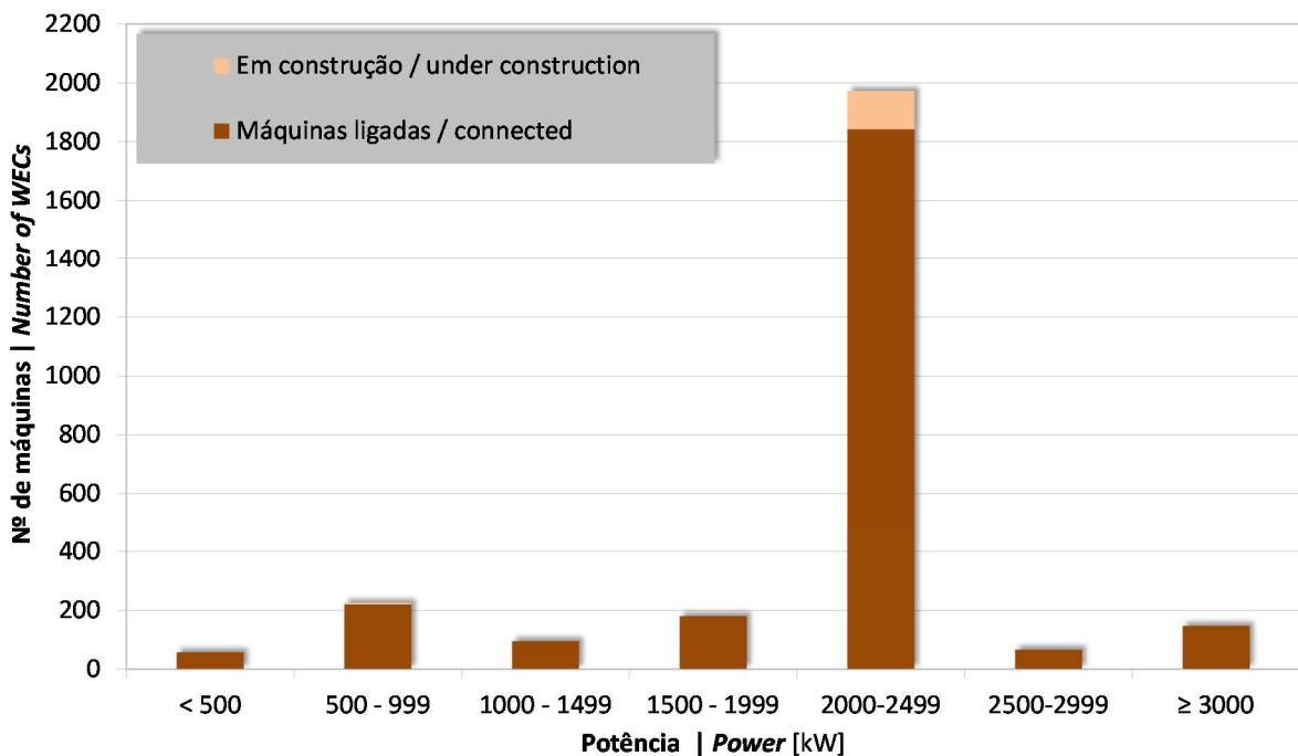
Figura 17: Número de aerogeradores por classes de potência 2015 Figure 17: Number of WECs and power classes 2015
