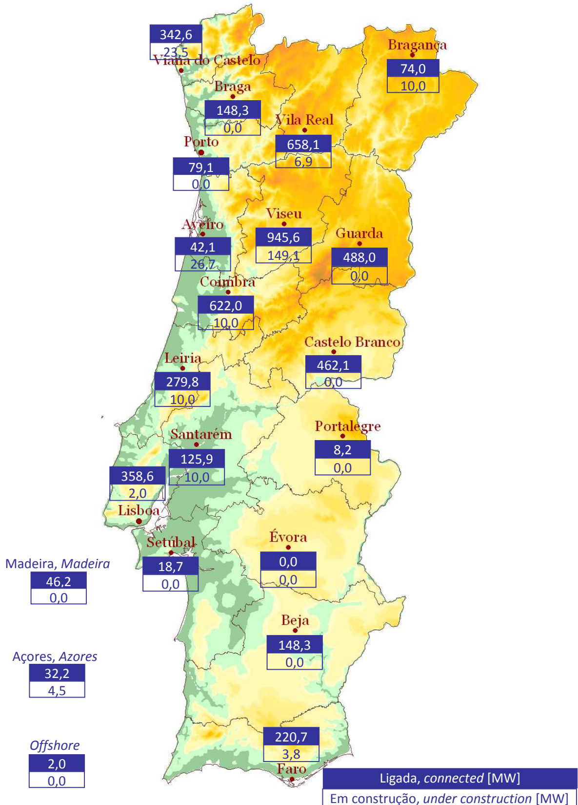
Figura 14: Potência Instalada por Distritos e Regiões Autónomas 2015 Figure 14: Installed capacity per district and autonomous region 2015 – Portugal mainland
