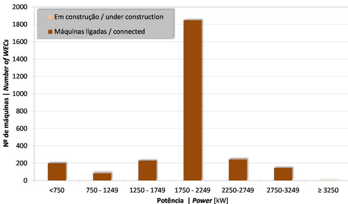
Figura 17: Número de aerogeradores por classes de potência 2016 Figure 17: Number of WECs and power classes 2016
