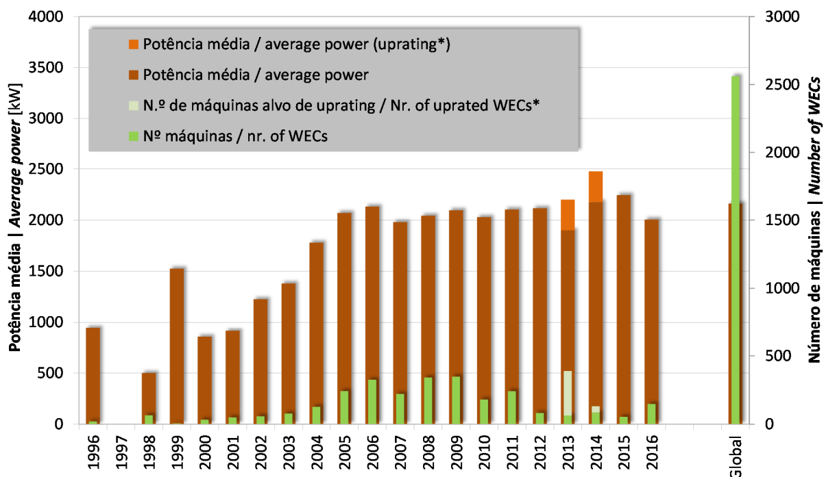
Figura 16: Número de aerogeradores e potência unitária média 1996-2016 Figure 16: Number of WECs and mean rated power 1996-2016
