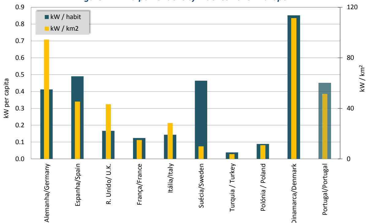
Figura 4: Índices de densidade 2018 - Europa Figure 4: Wind power density indexes 2018 - Europe
