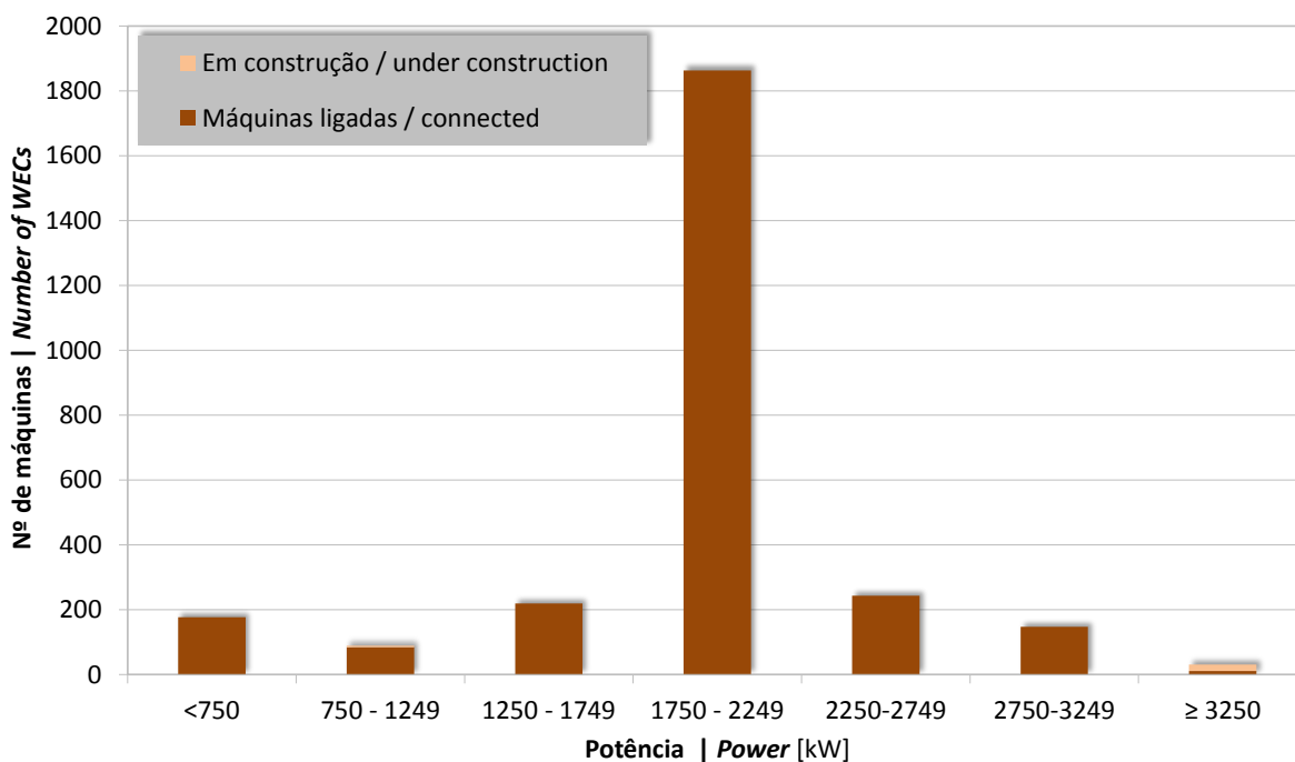
Figura 17: Número de aerogeradores por classes de potência 2018 Figure 17: Number of WECs and power classes 2018
