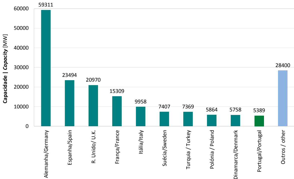
Figura 2: Potência capacidade geradora 2018 - Europa Figure 2: Installed capacity 2018 - Europe
