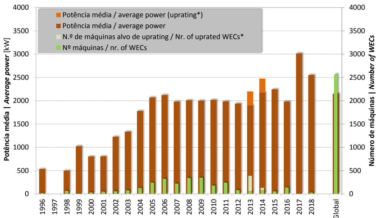
Figura 16: Número de aerogeradores e potência unitária média 1996-2018 Figure 16: Number of WECs and mean rated power 1996-2018
