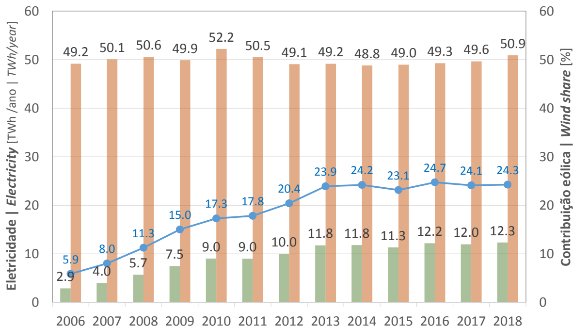
Figura 8: Geração eólica vs. Consumo de eletricidade 2018 Portugal Continental
