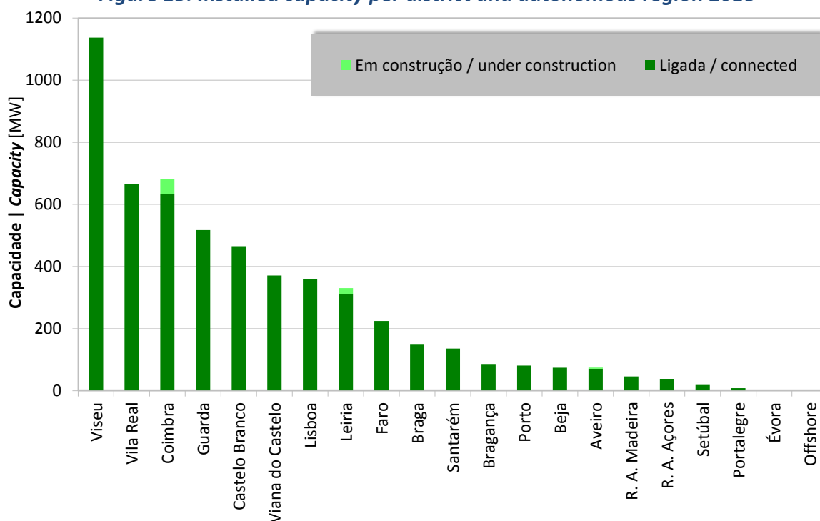
Figura 13: Potência Instalada por Distritos e Regiões Autónomas 2018 Figure 13: Installed capacity per district and autonomous region 2018
