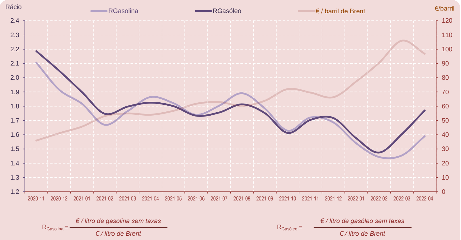
Evolução dos rácios R_{Gasóleo} e R_{Gasolina} (preços do litro de combustível / preço do litro de Brent)
